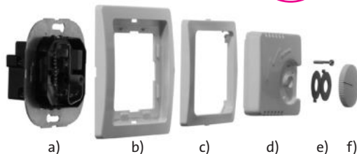
Montagebild Raumthermostat
